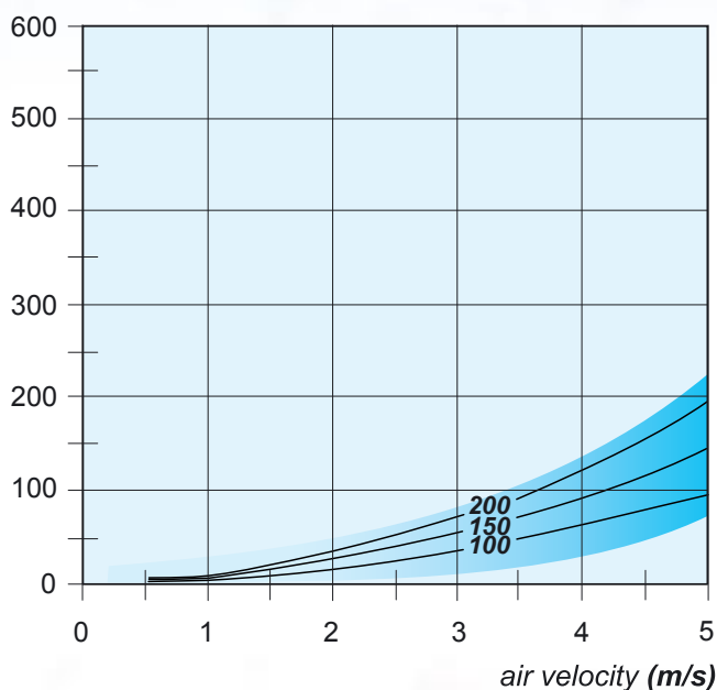
Pressure drop (Pa)
